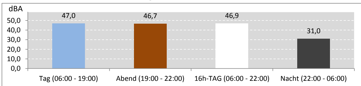
Abb. 7: LEQ bei Pistenbetriebsrichtung "westliche Winde" 250 Stunden im Messzeitraum
