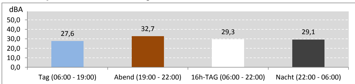
Abb. 9: LEQ bei Pistenbetriebsrichtung "östliche Winde" 98 Stunden im Messzeitraum
