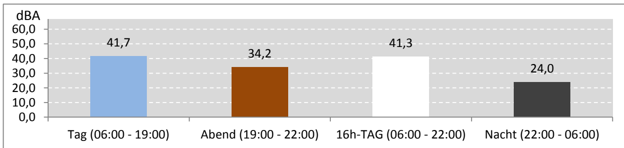
Abb. 9: LEQ bei Pistenbetriebsrichtung "östliche Winde" 104 Stunden im Messzeitraum
