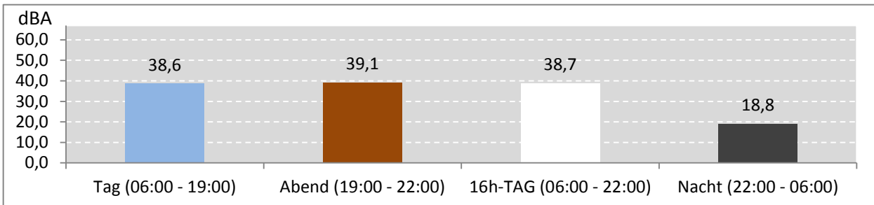
Abb. 6: LEQ für den gesamten Messzeitraum während der Messdauer (Gesamt: 575 Stunden)
