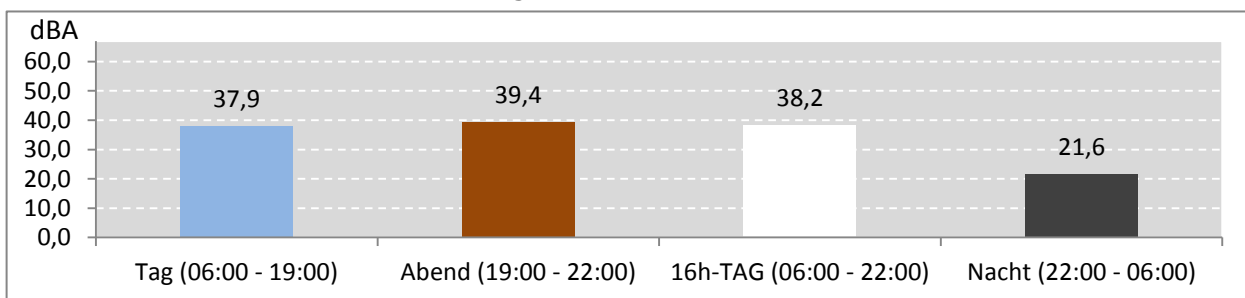
Abb. 7: LEQ bei Pistenbetriebsrichtung "westliche Winde" 316 Stunden im Messzeitraum
