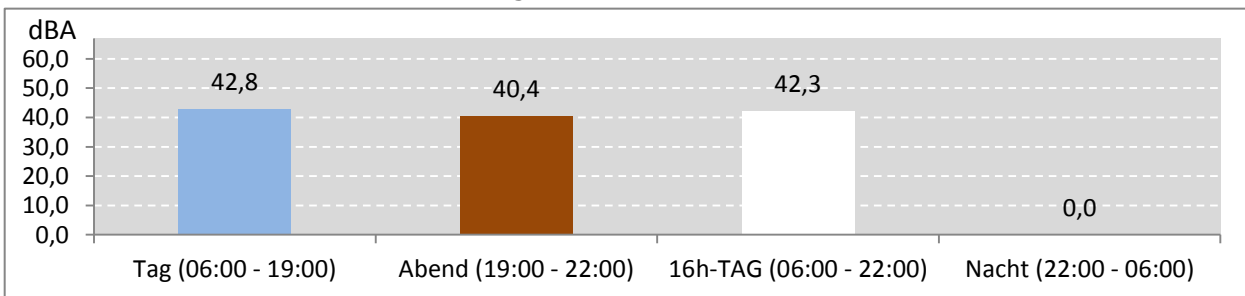
Abb. 8: LEQ bei Pistenbetriebsrichtung "Windstille" 135 Stunden im Messzeitraum
