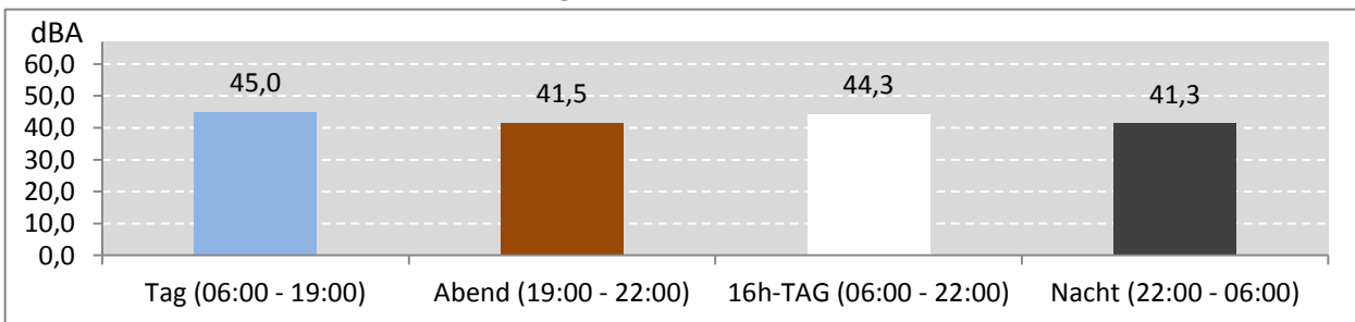
Abb. 8: LEQ bei Pistenbetriebsrichtung "Windstille" 86 Stunden im Messzeitraum
