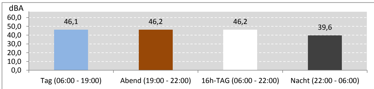
Abb. 7: LEQ bei Pistenbetriebsrichtung "westliche Winde" 285 Stunden im Messzeitraum
