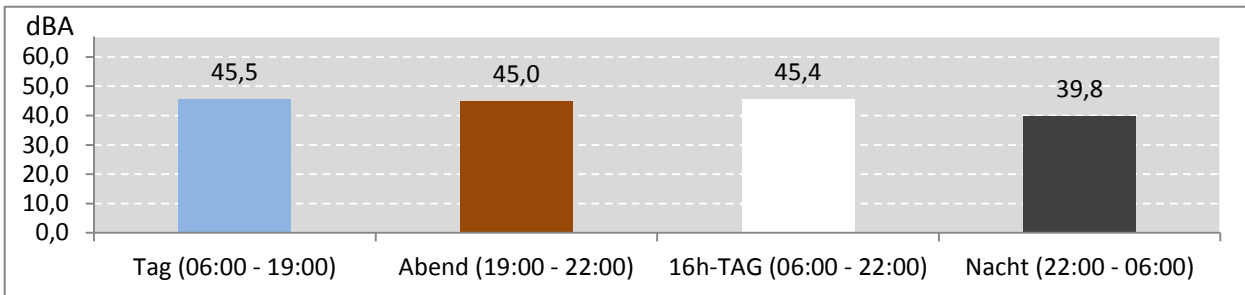
Abb. 6: LEQ für den gesamten Messzeitraum während der Messdauer (Gesamt: 463 Stunden)
