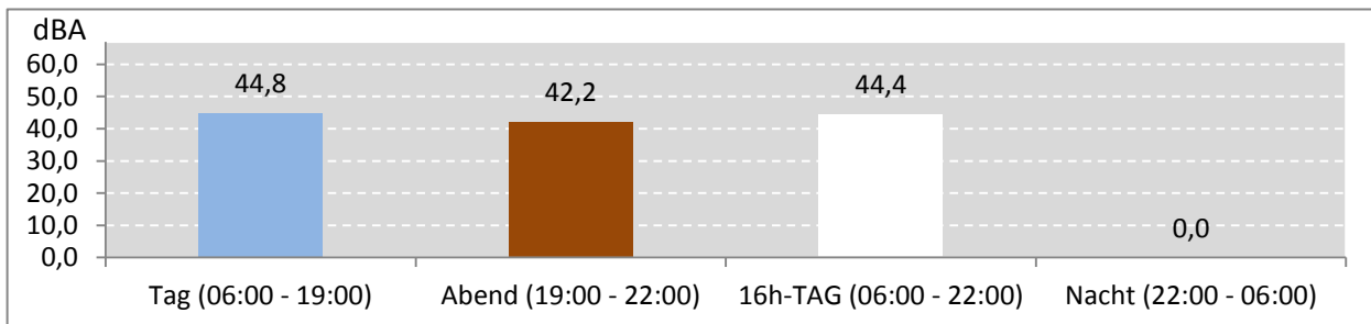
Abb. 7: LEQ bei Pistenbetriebsrichtung "westliche Winde" 370 Stunden im Messzeitraum
