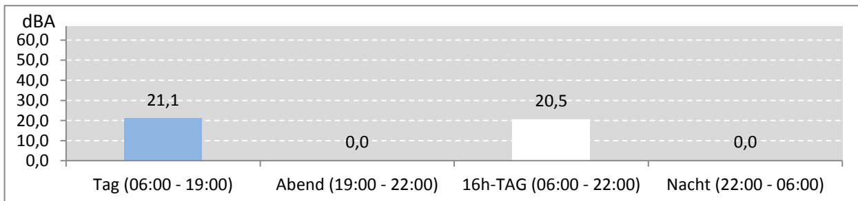
Abb. 9: LEQ bei Pistenbetriebsrichtung "östliche Winde" 25 Stunden im Messzeitraum
