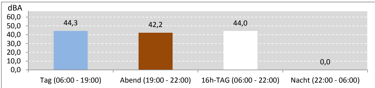
Abb. 6: LEQ für den gesamten Messzeitraum während der Messdauer (Gesamt: 483 Stunden)
