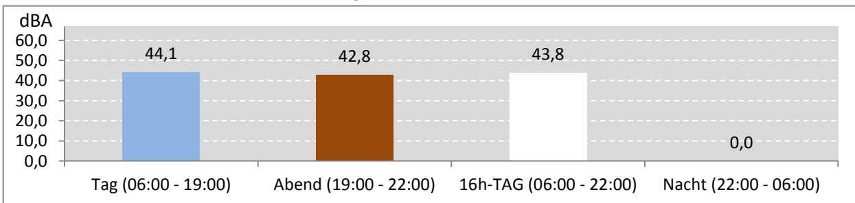
Abb. 8: LEQ bei Pistenbetriebsrichtung "Windstille" 88 Stunden im Messzeitraum
