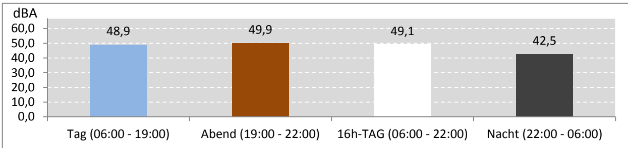
Abb. 6: LEQ für den gesamten Messzeitraum während der Messdauer (Gesamt: 455 Stunden)
