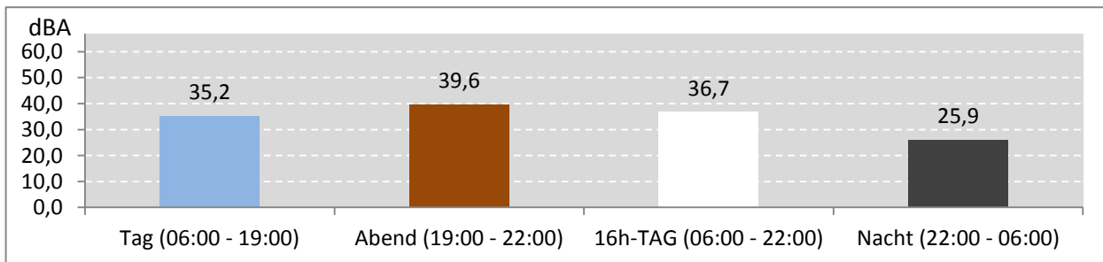
Abb. 9: LEQ bei Pistenbetriebsrichtung "östliche Winde" 43 Stunden im Messzeitraum
