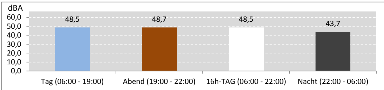
Abb. 6: LEQ für den gesamten Messzeitraum während der Messdauer (Gesamt: 505 Stunden)
