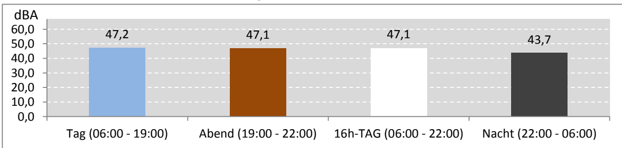
Abb. 8: LEQ bei Pistenbetriebsrichtung "Windstille" 126 Stunden im Messzeitraum
