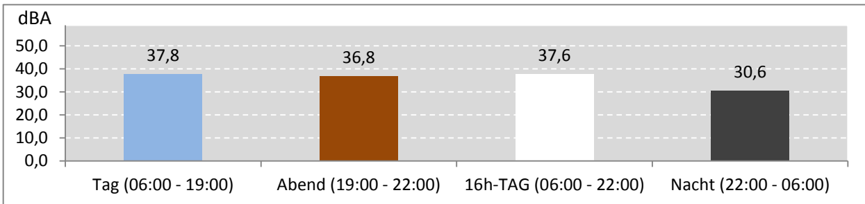
Abb. 6: LEQ für den gesamten Messzeitraum während der Messdauer (Gesamt: 430 Stunden)
