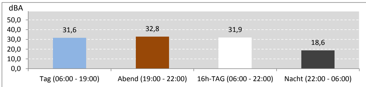
Abb. 7: LEQ bei Pistenbetriebsrichtung "westliche Winde" 205 Stunden im Messzeitraum
