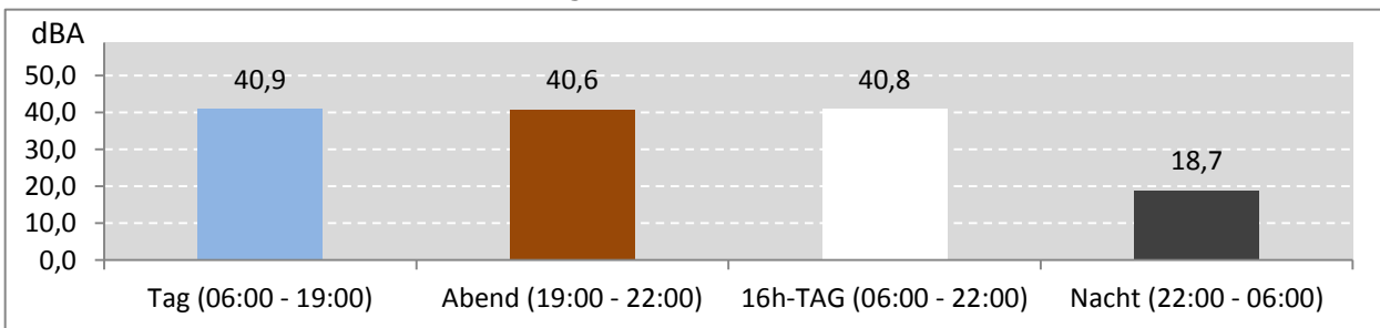
Abb. 8: LEQ bei Pistenbetriebsrichtung "Windstille" 102 Stunden im Messzeitraum
