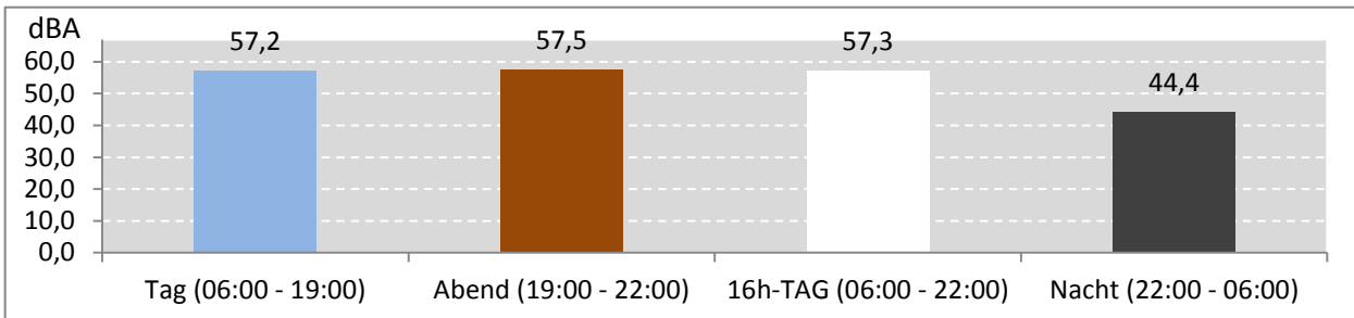
Abb. 6: LEQ für den gesamten Messzeitraum während der Messdauer (Gesamt: 569 Stunden)
