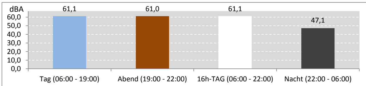
Abb. 9: LEQ bei Pistenbetriebsrichtung "östliche Winde" 183 Stunden im Messzeitraum
