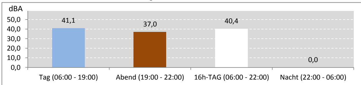
Abb. 8: LEQ bei Pistenbetriebsrichtung "Windstille" 89 Stunden im Messzeitraum
