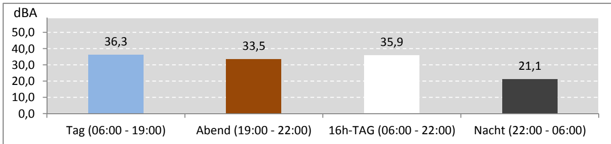
Abb. 6: LEQ für den gesamten Messzeitraum während der Messdauer (Gesamt: 448 Stunden)
