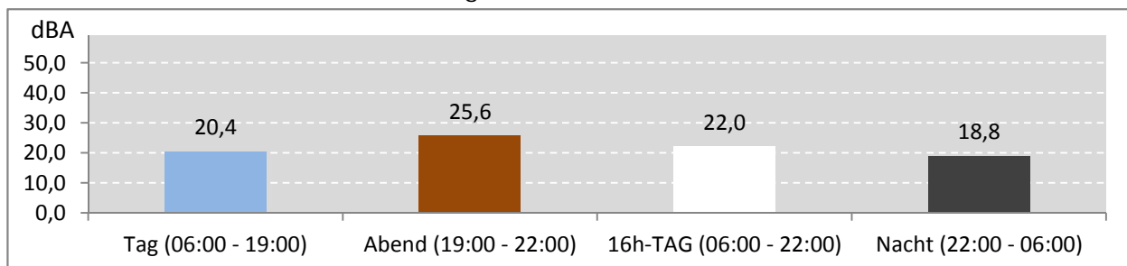
Abb. 9: LEQ bei Pistenbetriebsrichtung "östliche Winde" 233 Stunden im Messzeitraum
