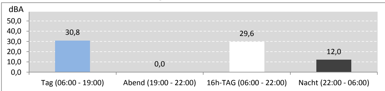
Abb. 8: LEQ bei Pistenbetriebsrichtung "Windstille" 82 Stunden im Messzeitraum
