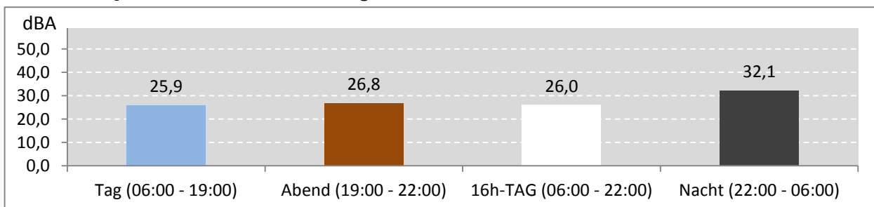
Abb. 9: LEQ bei Pistenbetriebsrichtung "östliche Winde" 264 Stunden im Messzeitraum
