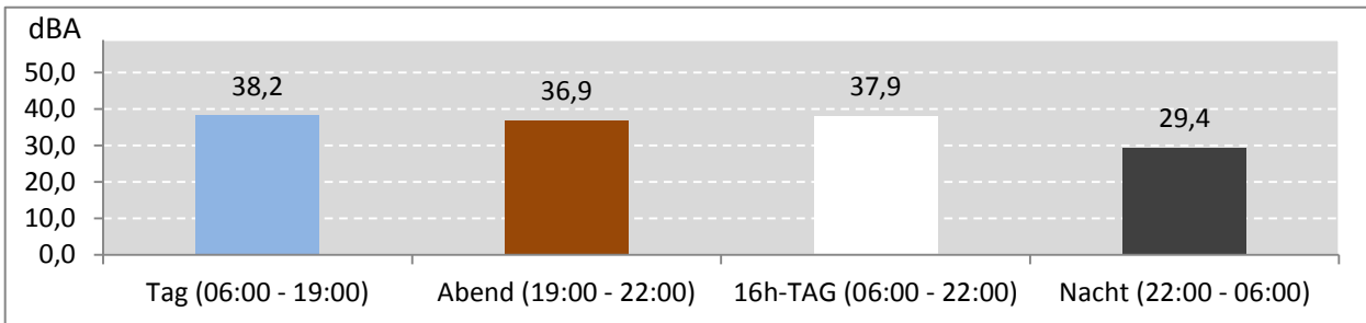
Abb. 6: LEQ für den gesamten Messzeitraum während der Messdauer (Gesamt: 472 Stunden)
