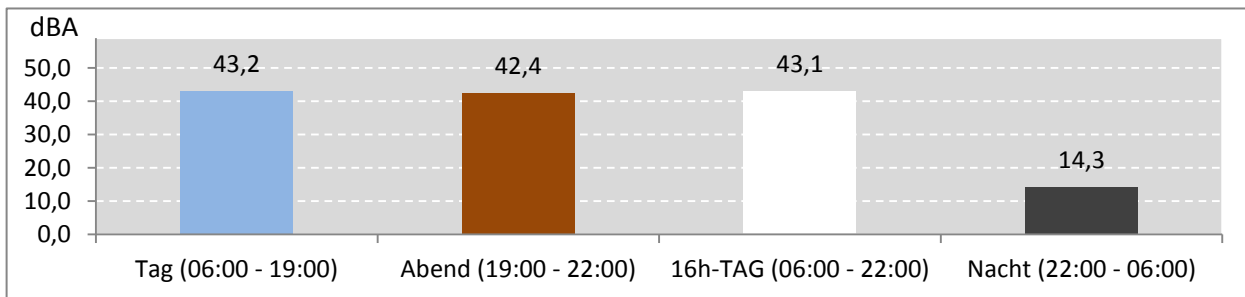
Abb. 7: LEQ bei Pistenbetriebsrichtung "westliche Winde" 126 Stunden im Messzeitraum
