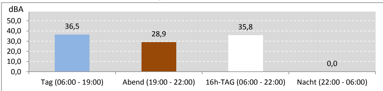
Abb. 8: LEQ bei Pistenbetriebsrichtung "Windstille" 157 Stunden im Messzeitraum
