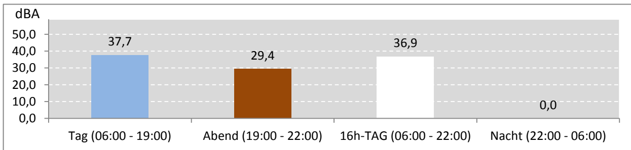
Abb. 7: LEQ bei Pistenbetriebsrichtung "westliche Winde" 198 Stunden im Messzeitraum
