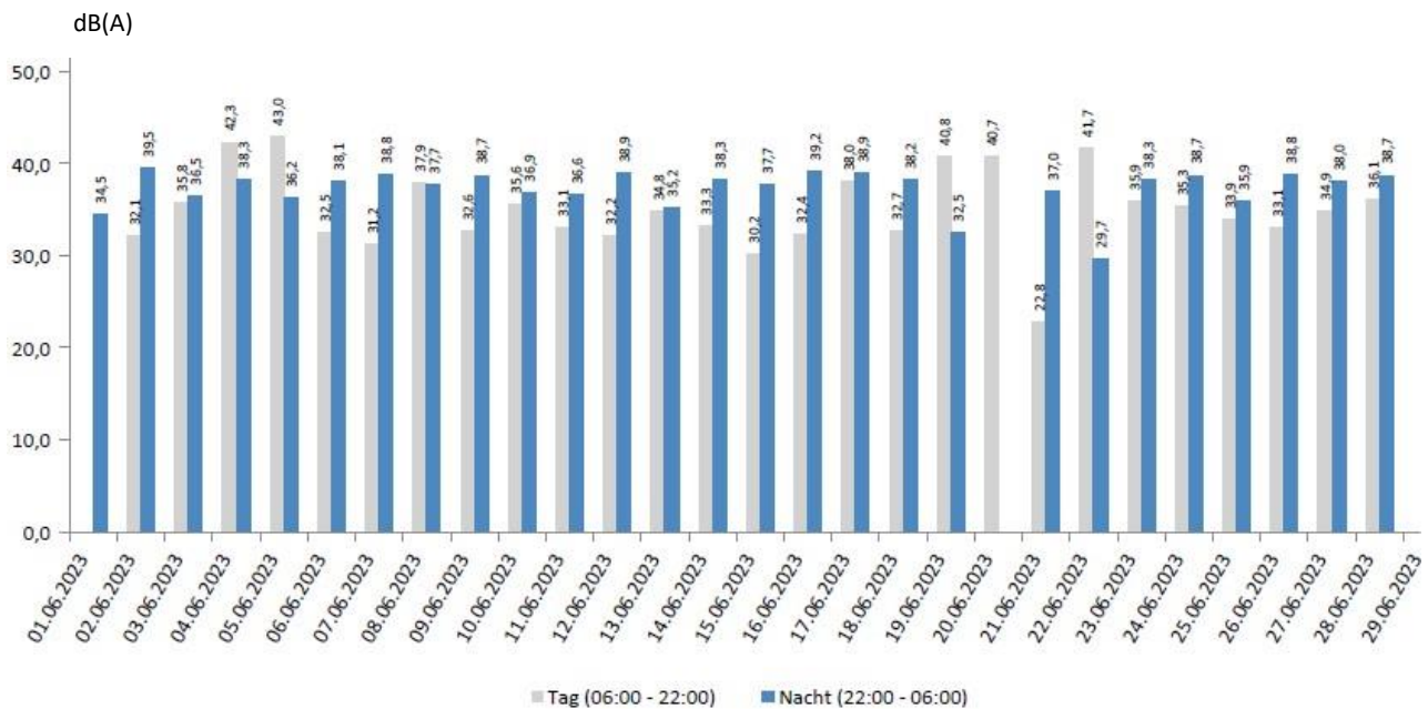
Abb.10: LEQ für Flugverkehr über den Messzeitraum
