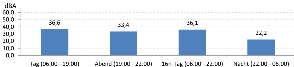
Abb. 9: LEQ bei Pistenbetriebsrichtung "östliche Winde" 170 Stunden im Messzeitraum
