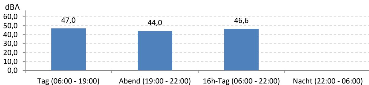
Abb. 7: LEQ bei Pistenbetriebsrichtung "westliche Winde" 394 Stunden im Messzeitraum
