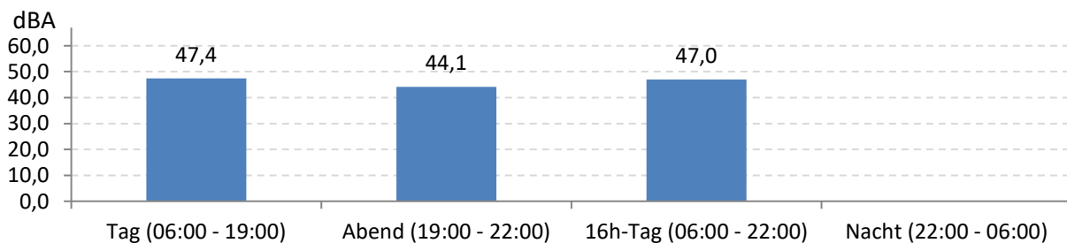
Abb. 8: LEQ bei Pistenbetriebsrichtung "Windstille" 156 Stunden im Messzeitraum
