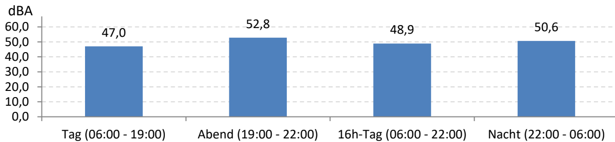
Abb. 7: LEQ bei Pistenbetriebsrichtung "westliche Winde" 436 Stunden im Messzeitraum
