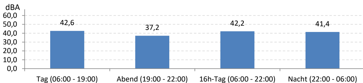
Abb. 9: LEQ bei Pistenbetriebsrichtung "östliche Winde" 171 Stunden im Messzeitraum
