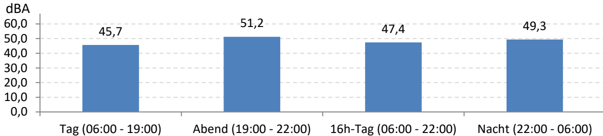
Abb. 6: LEQ für den gesamten Messzeitraum während der Messdauer (Gesamt: 791 Stunden)
