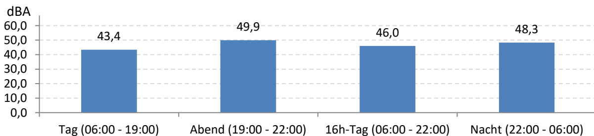
Abb. 8: LEQ bei Pistenbetriebsrichtung "Windstille" 184 Stunden im Messzeitraum
