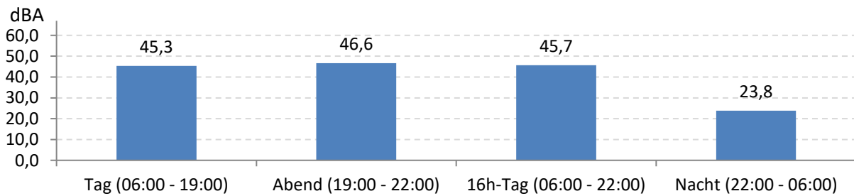
Abb. 8: LEQ bei Pistenbetriebsrichtung "Windstille" 220 Stunden im Messzeitraum
