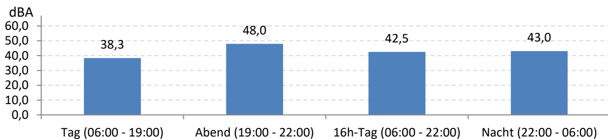
Abb. 9: LEQ bei Pistenbetriebsrichtung "östliche Winde" 215 Stunden im Messzeitraum
