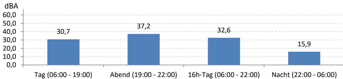
Abb. 7: LEQ bei Pistenbetriebsrichtung "westliche Winde" 309 Stunden im Messzeitraum
