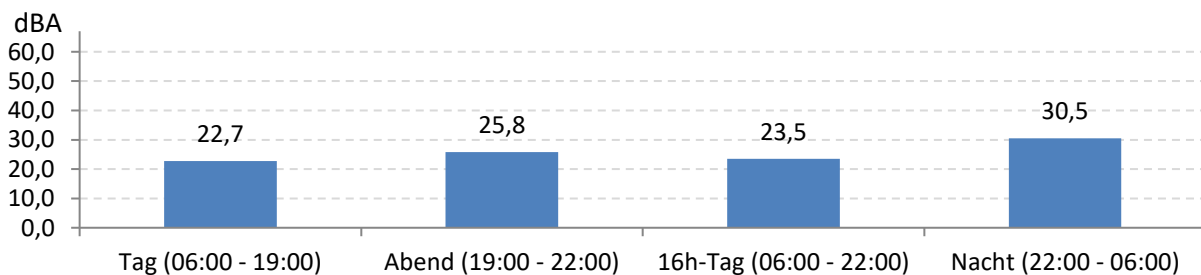
Abb. 8: LEQ bei Pistenbetriebsrichtung "Windstille" 198 Stunden im Messzeitraum
