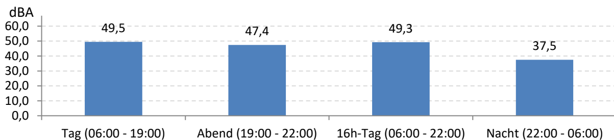
Abb. 9: LEQ bei Pistenbetriebsrichtung "östliche Winde" 87 Stunden im Messzeitraum
