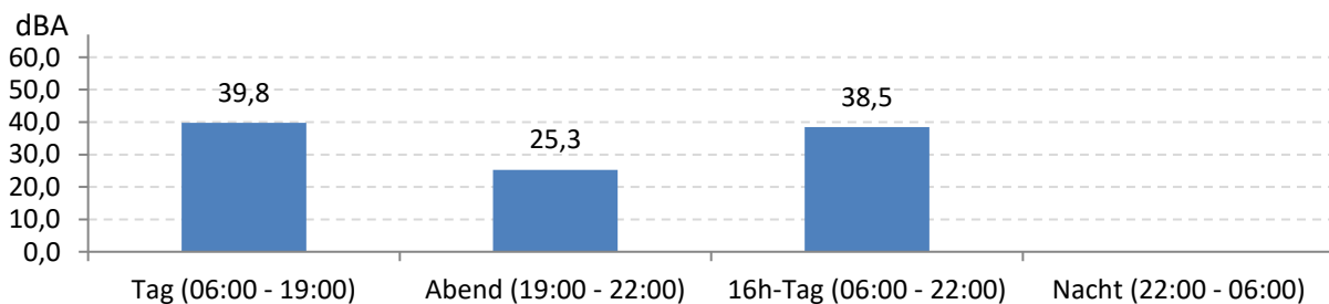
Abb. 8: LEQ bei Pistenbetriebsrichtung "Windstille" 183 Stunden im Messzeitraum
