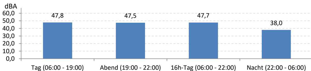
Abb. 9: LEQ bei Pistenbetriebsrichtung "östliche Winde" 87 Stunden im Messzeitraum
