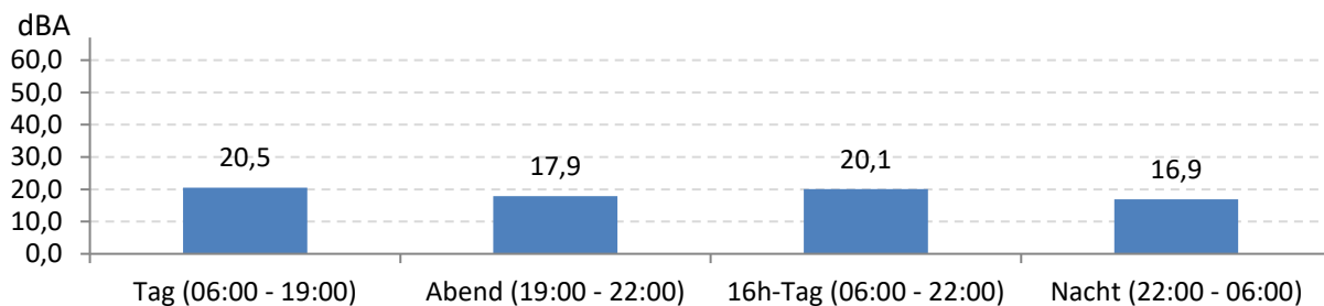
Abb. 7: LEQ bei Pistenbetriebsrichtung "westliche Winde" 450 Stunden im Messzeitraum
