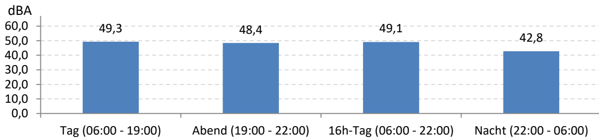
Abb. 7: LEQ bei Pistenbetriebsrichtung "westliche Winde" 487 Stunden im Messzeitraum
