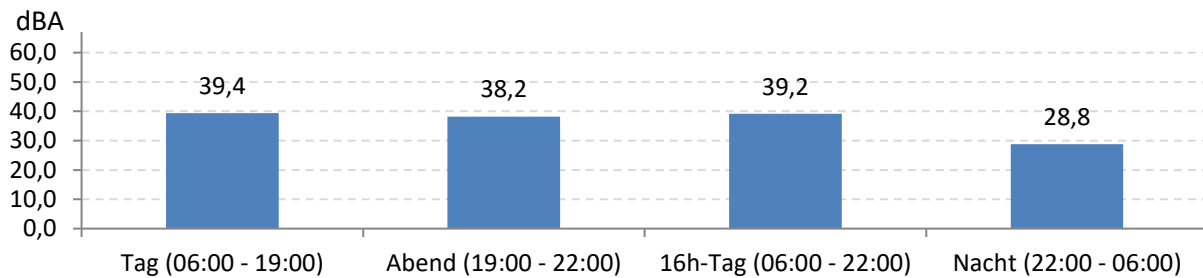
Abb. 7: LEQ bei Pistenbetriebsrichtung "westliche Winde" 379 Stunden im Messzeitraum
