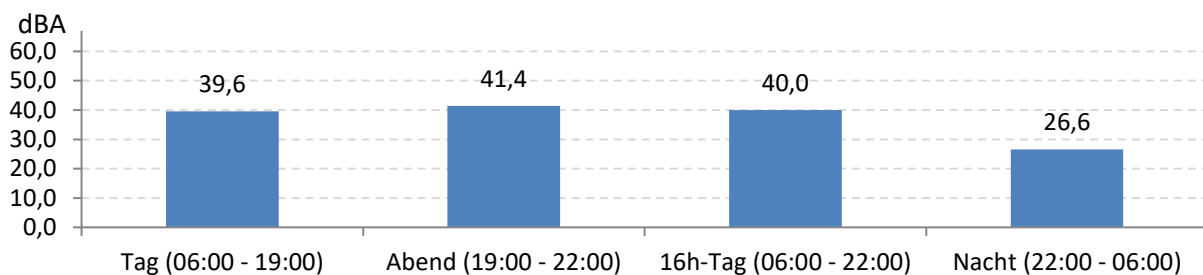
Abb. 9: LEQ bei Pistenbetriebsrichtung "östliche Winde" 200 Stunden im Messzeitraum
