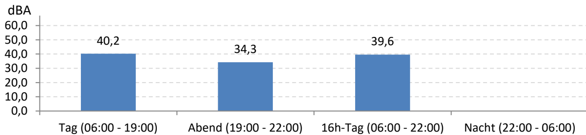
Abb. 7: LEQ bei Pistenbetriebsrichtung "westliche Winde" 387 Stunden im Messzeitraum
