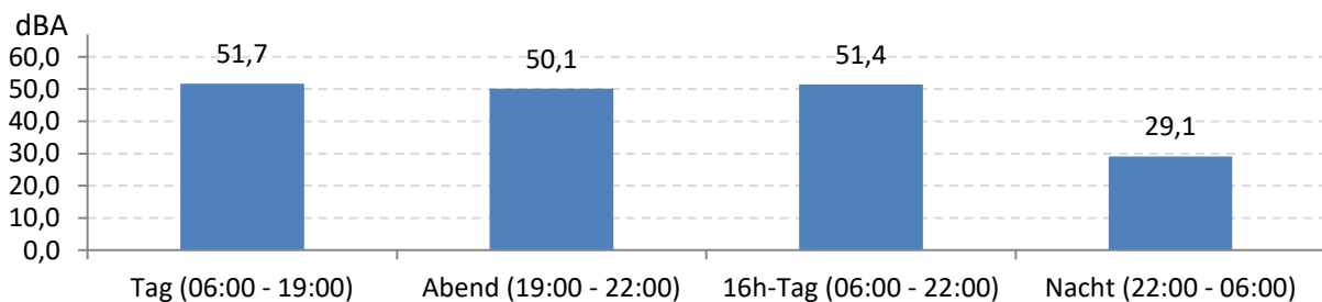
Abb. 8: LEQ bei Pistenbetriebsrichtung "Windstille" 231 Stunden im Messzeitraum
