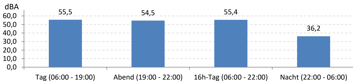
Abb. 7: LEQ bei Pistenbetriebsrichtung "westliche Winde" 412 Stunden im Messzeitraum
