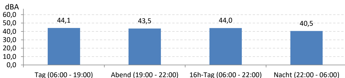
Abb. 9: LEQ bei Pistenbetriebsrichtung "östliche Winde" 154 Stunden im Messzeitraum
