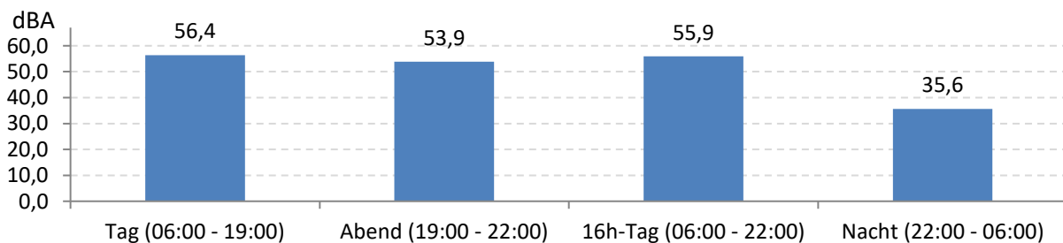
Abb. 8: LEQ bei Pistenbetriebsrichtung "Windstille" 250 Stunden im Messzeitraum
