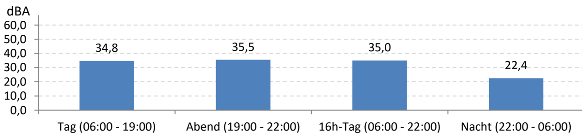
Abb. 8: LEQ bei Pistenbetriebsrichtung "Windstille"
