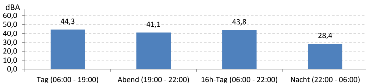
Abb. 9: LEQ bei Pistenbetriebsrichtung "östliche Winde"
