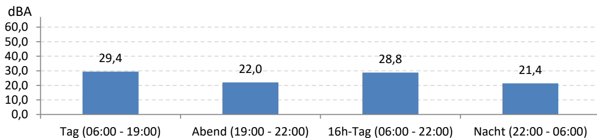
Abb. 7: LEQ bei Pistenbetriebsrichtung "westliche Winde"
