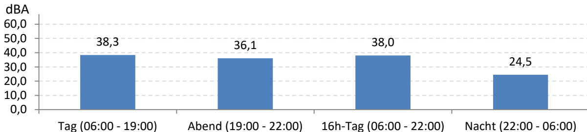
Abb. 6: LEQ für den gesamten Messzeitraum während der Messdauer (Gesamt: 624 Stunden)
