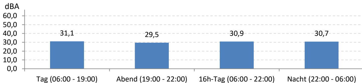
Abb. 7: LEQ bei Pistenbetriebsrichtung "westliche Winde" 433 Stunden im Messzeitraum
