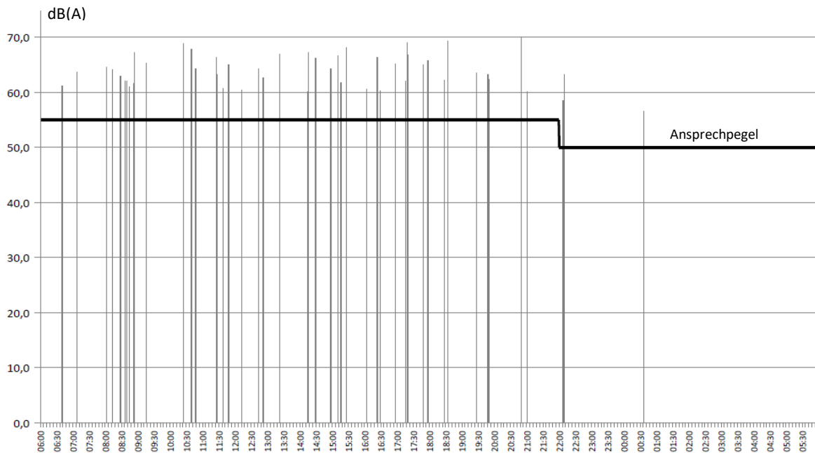
Abb. 13: Verteilung des Maximalpegels bei östlichen Winden
