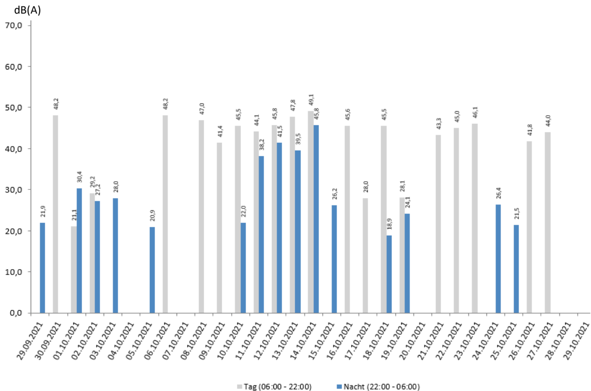
Abb. 11: Verlauf der über den Meßzeitraum gemittelten Stunden-LEQs für Flugverkehr
