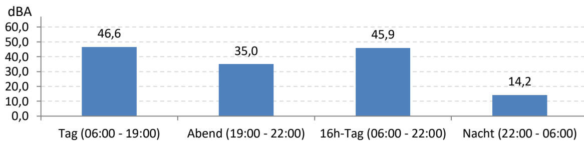
Abb. 7: LEQ bei Pistenbetriebsrichtung "westliche Winde" 308 Stunden im Messzeitraum
