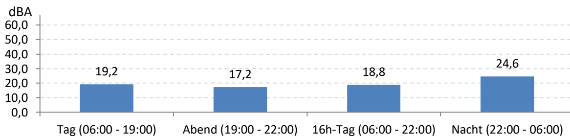
Abb. 9: LEQ bei Pistenbetriebsrichtung "östliche Winde" 321 Stunden im Messzeitraum
