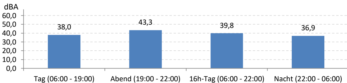
Abb. 8: LEQ bei Pistenbetriebsrichtung "Windstille" 188 Stunden im Messzeitraum
