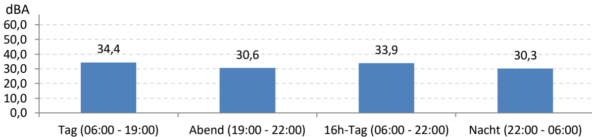
Abb. 6: LEQ für den gesamten Messzeitraum während der Messdauer (Gesamt: 744 Stunden)
