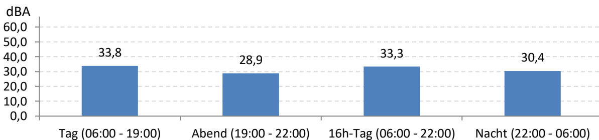
Abb. 7: LEQ bei Pistenbetriebsrichtung "westliche Winde" 398 Stunden im Messzeitraum
