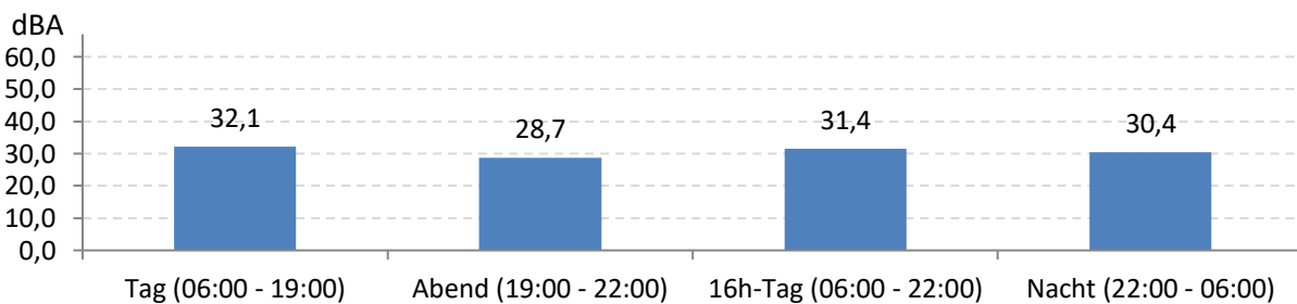
Abb. 8: LEQ bei Pistenbetriebsrichtung "Windstille" 244 Stunden im Messzeitraum
