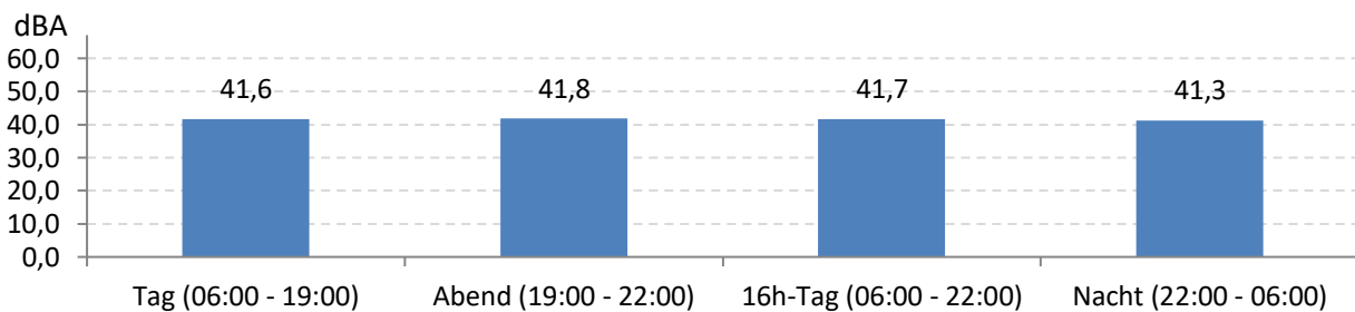
Abb. 8: LEQ bei Pistenbetriebsrichtung "Windstille" 129 Stunden im Messzeitraum
