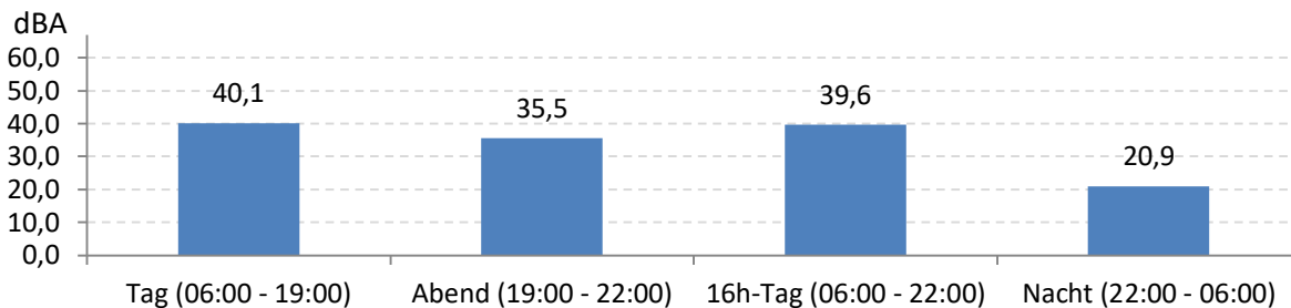
Abb. 7: LEQ bei Pistenbetriebsrichtung "westliche Winde" 390 Stunden im Messzeitraum
