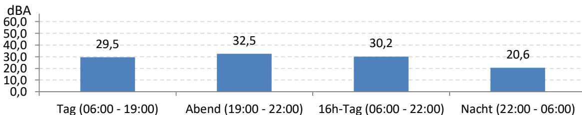
Abb. 9: LEQ bei Pistenbetriebsrichtung "östliche Winde" 173 Stunden im Messzeitraum
