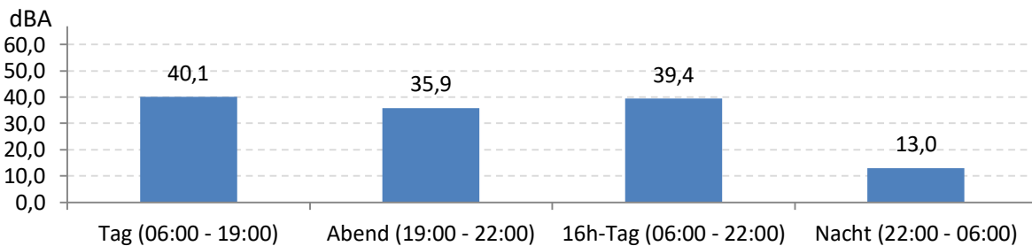
Abb. 8: LEQ bei Pistenbetriebsrichtung "Windstille" 181 Stunden im Messzeitraum
