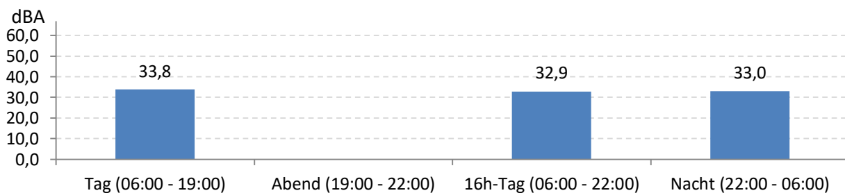
Abb. 9: LEQ bei Pistenbetriebsrichtung "östliche Winde" 173 Stunden im Messzeitraum
