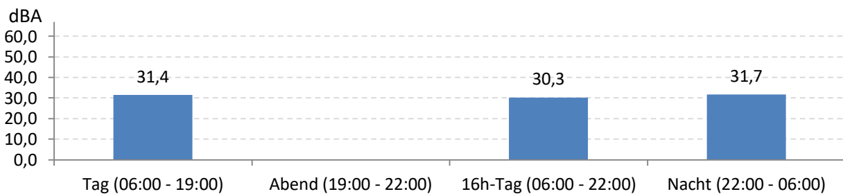
Abb. 8: LEQ bei Pistenbetriebsrichtung "Windstille" 181 Stunden im Messzeitraum
