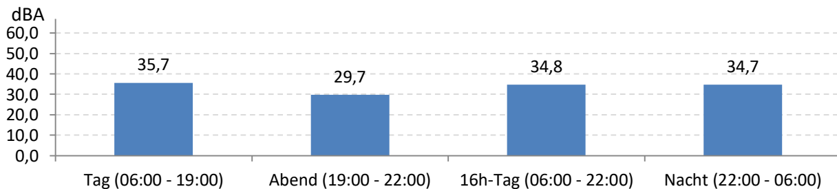
Abb. 9: LEQ bei Pistenbetriebsrichtung "östliche Winde" 206 Stunden im Messzeitraum
