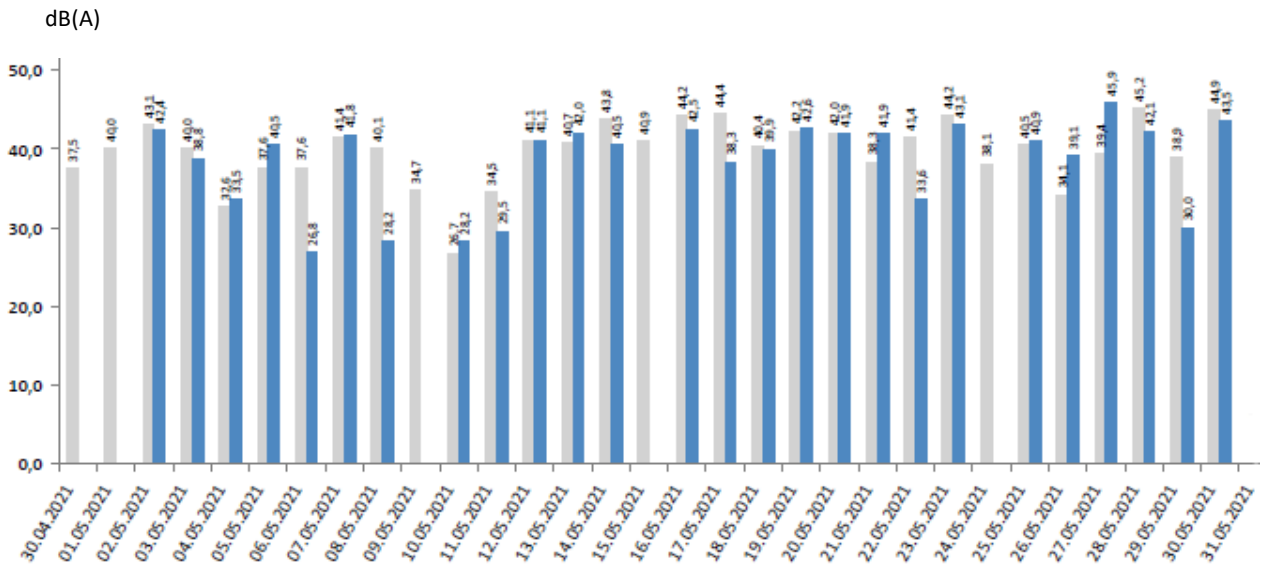
Abb.10: LEQ für Flugverkehr über den Messzeitraum
