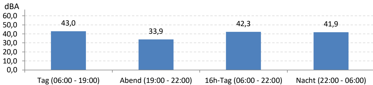
Abb. 7: LEQ bei Pistenbetriebsrichtung "westliche Winde" 463 Stunden im Messzeitraum
