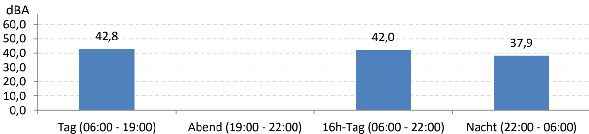
Abb. 8: LEQ bei Pistenbetriebsrichtung "Windstille" 99 Stunden im Messzeitraum
