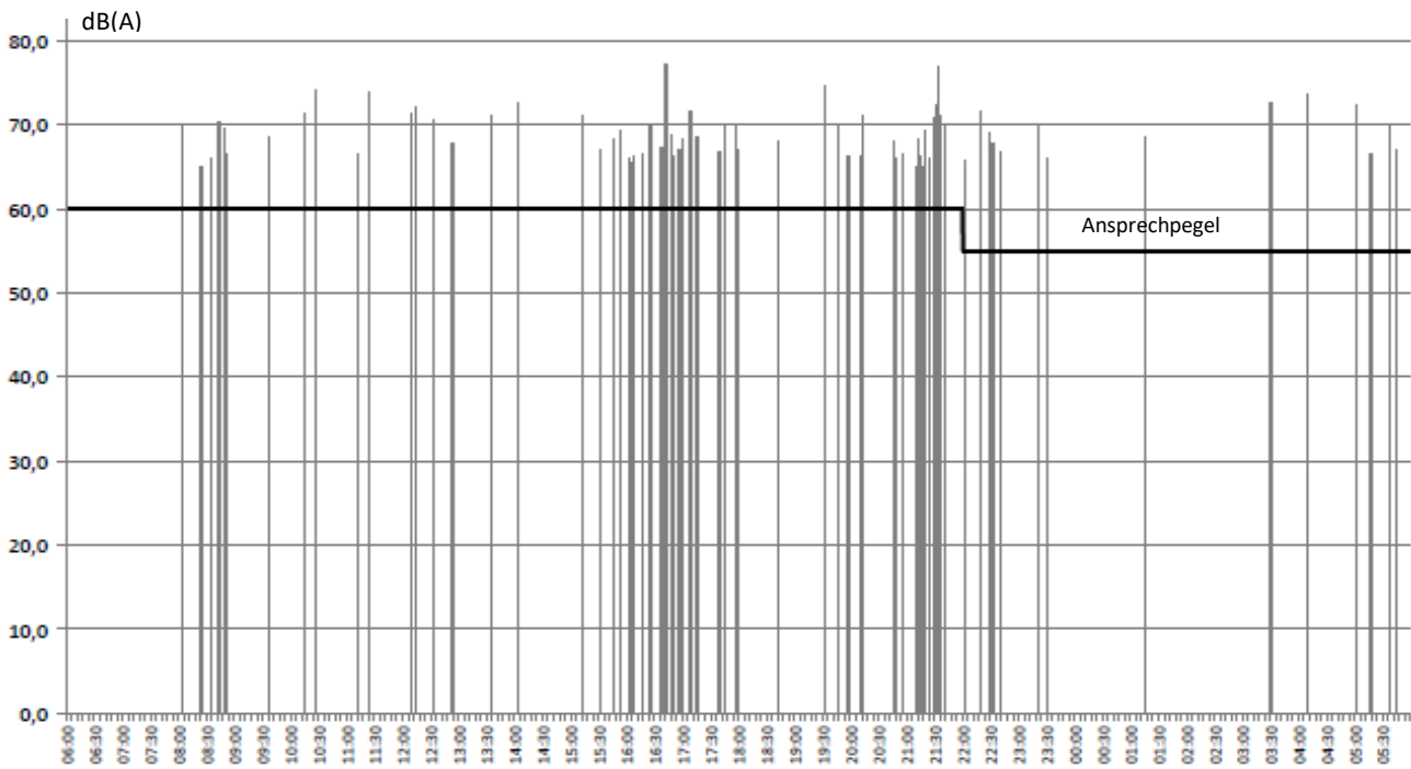
Abb. 13: Verteilung des Maximalpegels bei östlichen Winden
