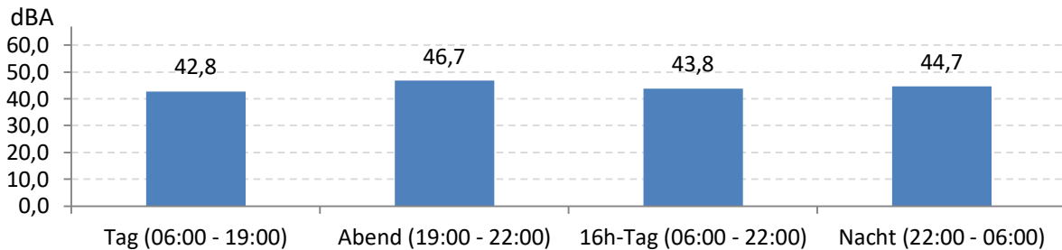
Abb. 6: LEQ für den gesamten Messzeitraum während der Messdauer (Gesamt: 887 Stunden)
