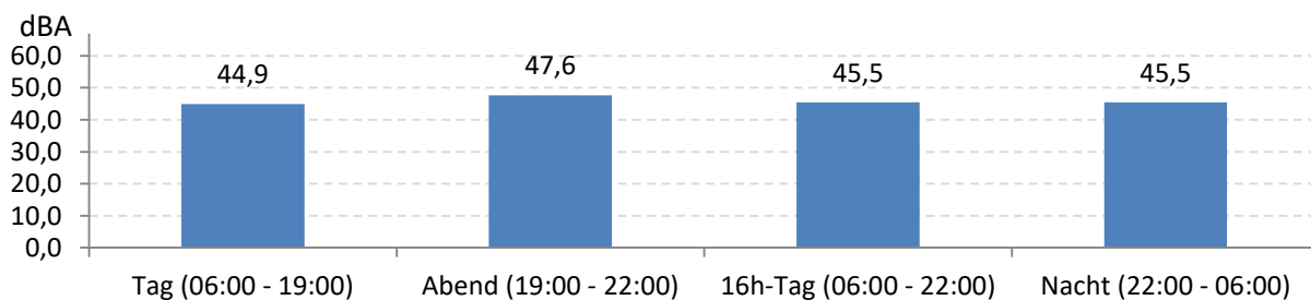
Abb. 9: LEQ bei Pistenbetriebsrichtung "östliche Winde" 102 Stunden im Messzeitraum
