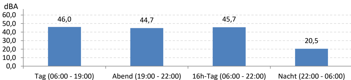
Abb. 8: LEQ bei Pistenbetriebsrichtung "Windstille" 213 Stunden im Messzeitraum
