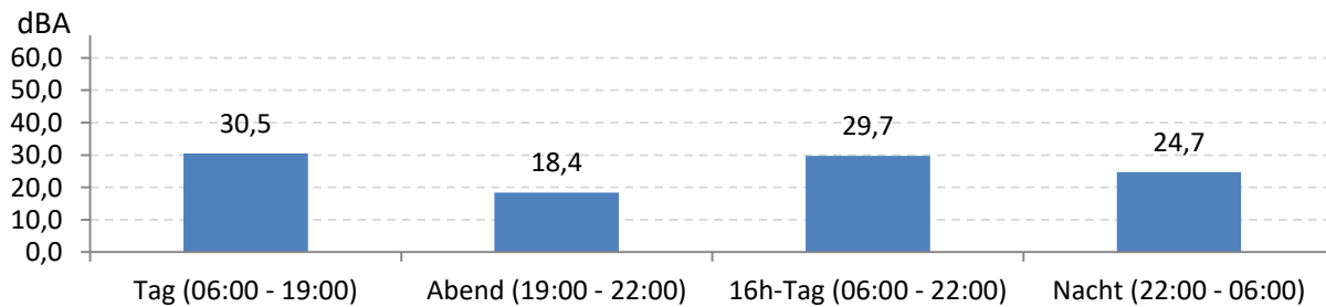
Abb. 7: LEQ bei Pistenbetriebsrichtung "westliche Winde" 429 Stunden im Messzeitraum
