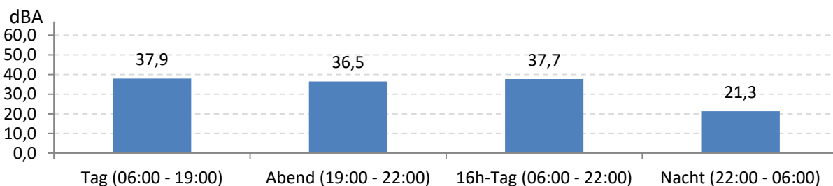
Abb. 9: LEQ bei Pistenbetriebsrichtung "östliche Winde" 147 Stunden im Messzeitraum
