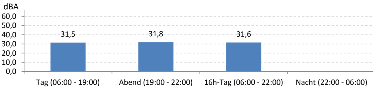
Abb. 7: LEQ bei Pistenbetriebsrichtung "westliche Winde" 464 Stunden im Messzeitraum
