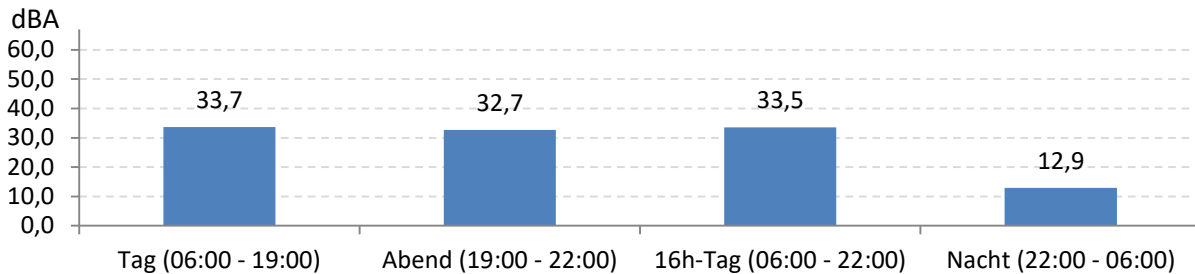
Abb. 6: LEQ für den gesamten Messzeitraum während der Messdauer (Gesamt: 816 Stunden)
