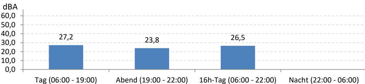
Abb. 8: LEQ bei Pistenbetriebsrichtung "Windstille" 205 Stunden im Messzeitraum
