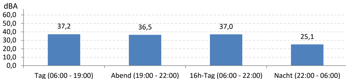
Abb. 6: LEQ für den gesamten Messzeitraum während der Messdauer (Gesamt: 768 Stunden)
