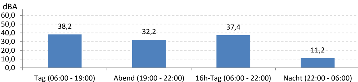
Abb. 8: LEQ bei Pistenbetriebsrichtung "Windstille" 689 Stunden im Messzeitraum
