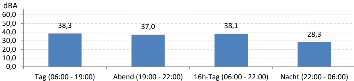
Abb. 6: LEQ für den gesamten Messzeitraum während der Messdauer (Gesamt: 2903 Stunden)
