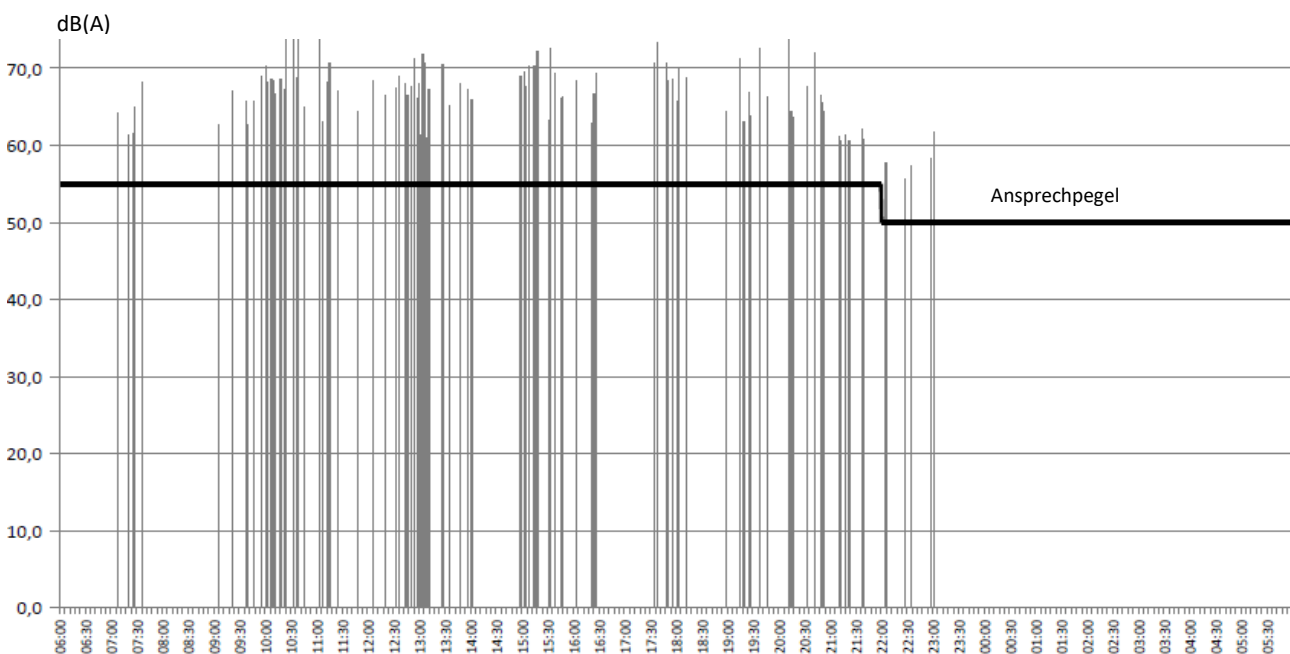
Abb. 13: Verteilung des Maximalpegels bei östlichen Winden
