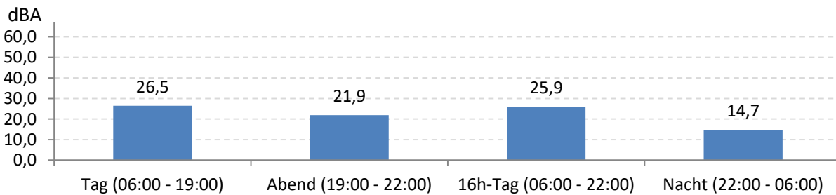
Abb. 7: LEQ bei Pistenbetriebsrichtung "westliche Winde" 1769 Stunden im Messzeitraum
