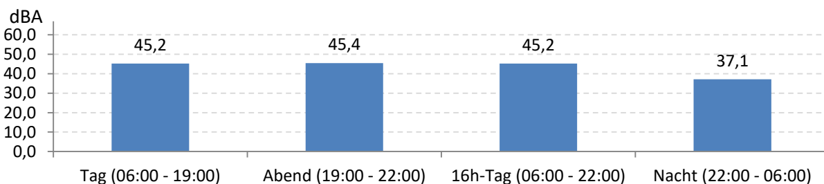
Abb. 9: LEQ bei Pistenbetriebsrichtung "östliche Winde" 445 Stunden im Messzeitraum
